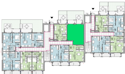
Aukšto planas
